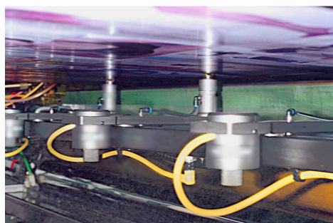
Barra del ABD estirando la anchura de la banda sin contacto mediante presión de aire.
