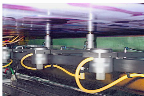
Zonder contact met de baan corrigeert de ABD register-nozzle de fan-out over de hele baan
