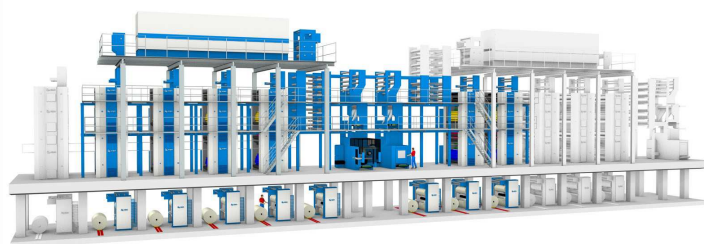
Jordan Press' KBA Commander met zes torens, twee vouwers en een droger.
